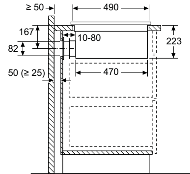
Vista laterale
