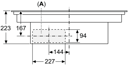
Vista frontale
