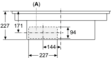
Vista frontale
